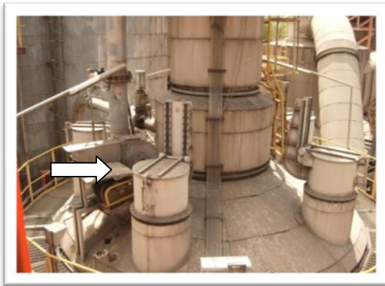
Deflagration vent door
